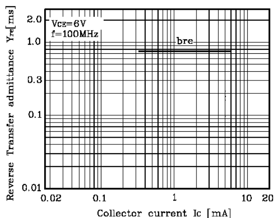
Fig. 9 I_C - Y_{re}
